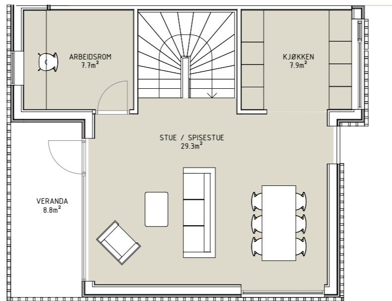
PLAN 2 1 : 100
