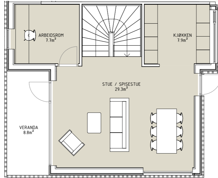
PLAN 2 1 : 100
