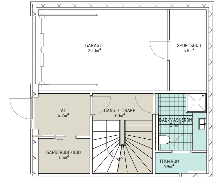
PLAN U 1 : 100
