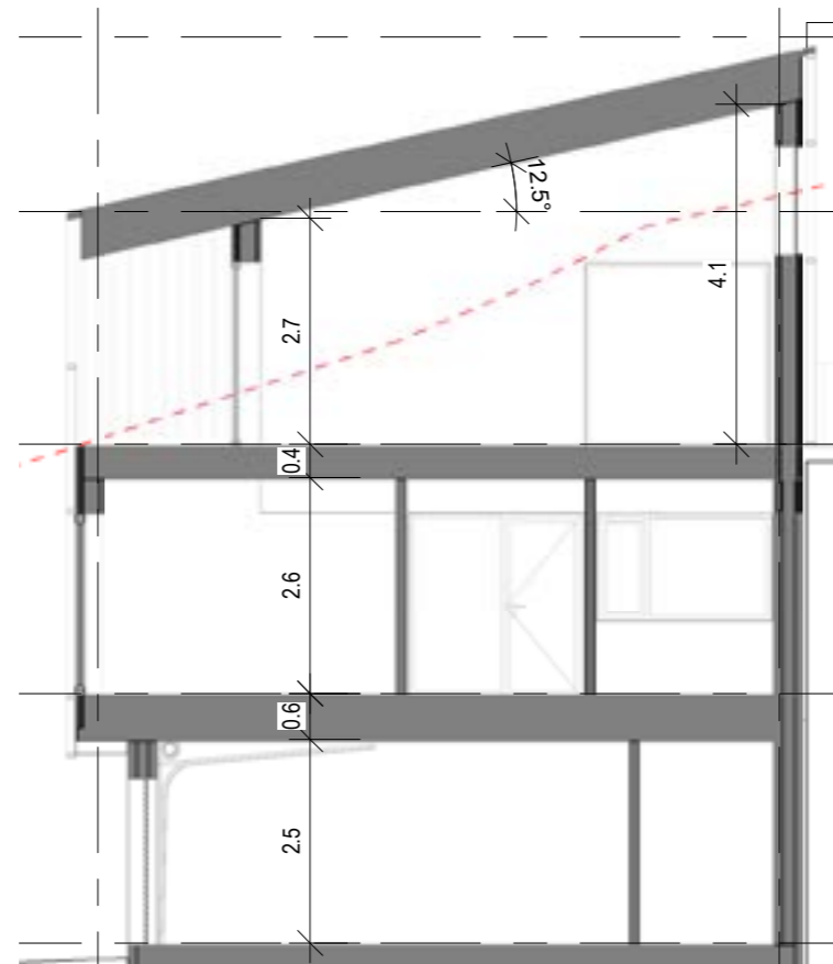
Snitt
