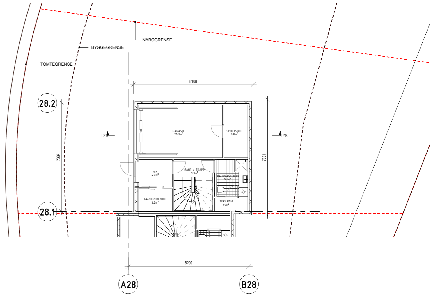
PLAN U 1 : 100
