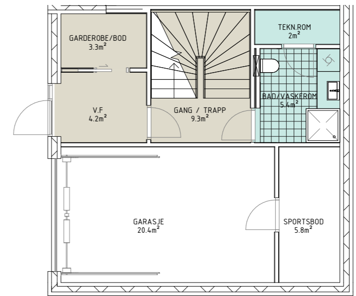
PLAN U 1 : 100
