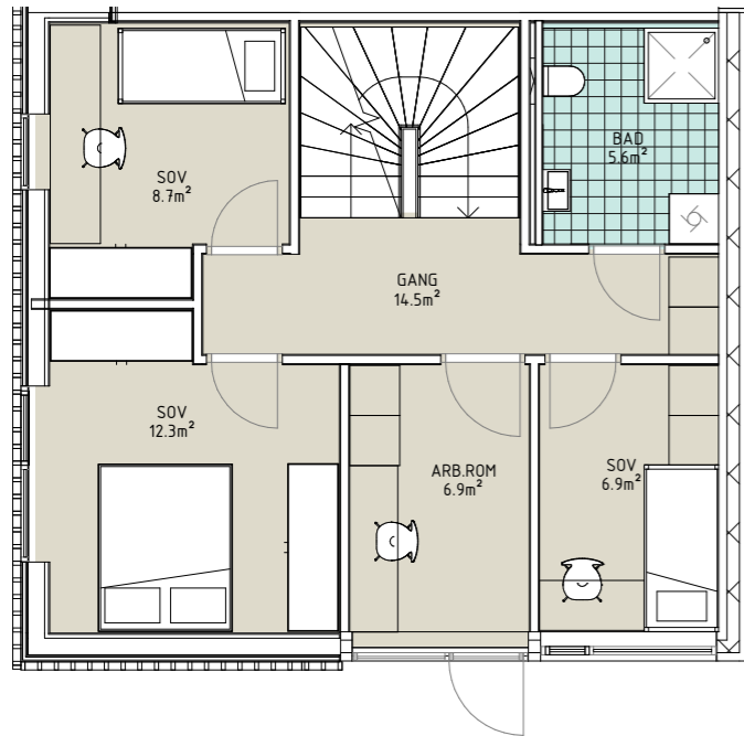
PLAN 1 1 : 100
