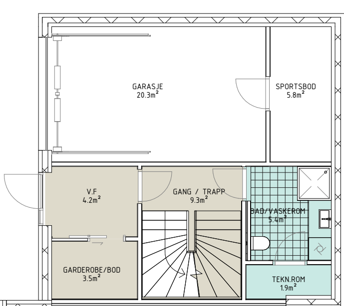
PLAN U 1 : 100
