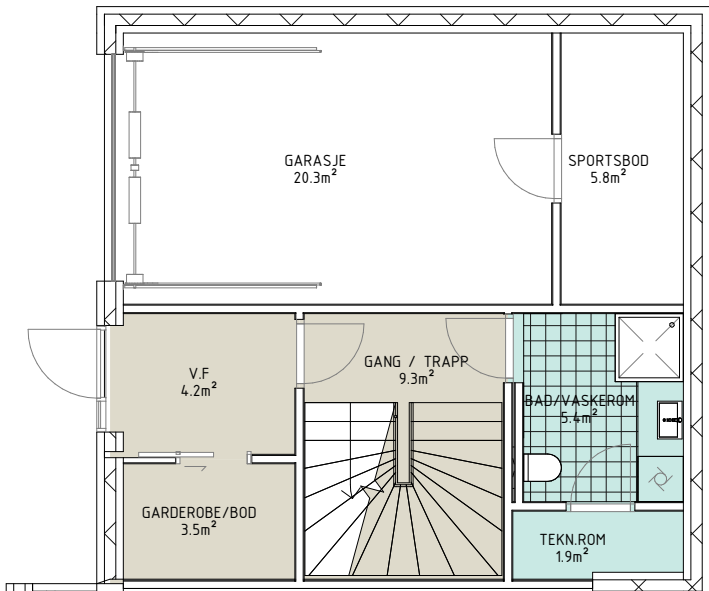
PLAN U 1 : 100
