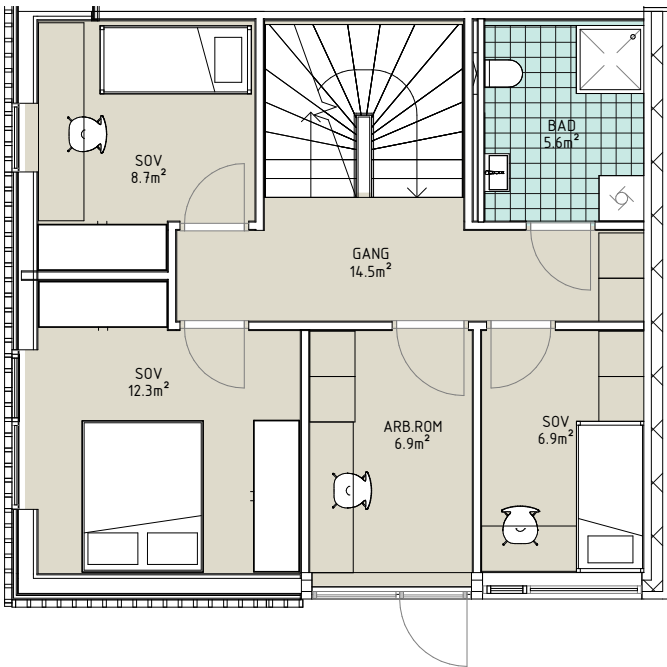
PLAN 1 1 : 100
