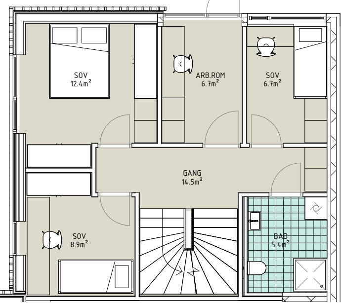
PLAN 1 1 : 100
