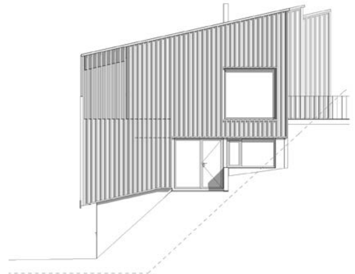
Fasader Sør
