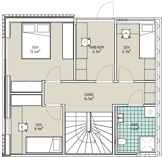
PLAN 1 1 : 100
