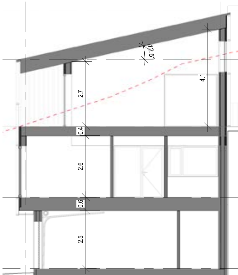
Snitt
