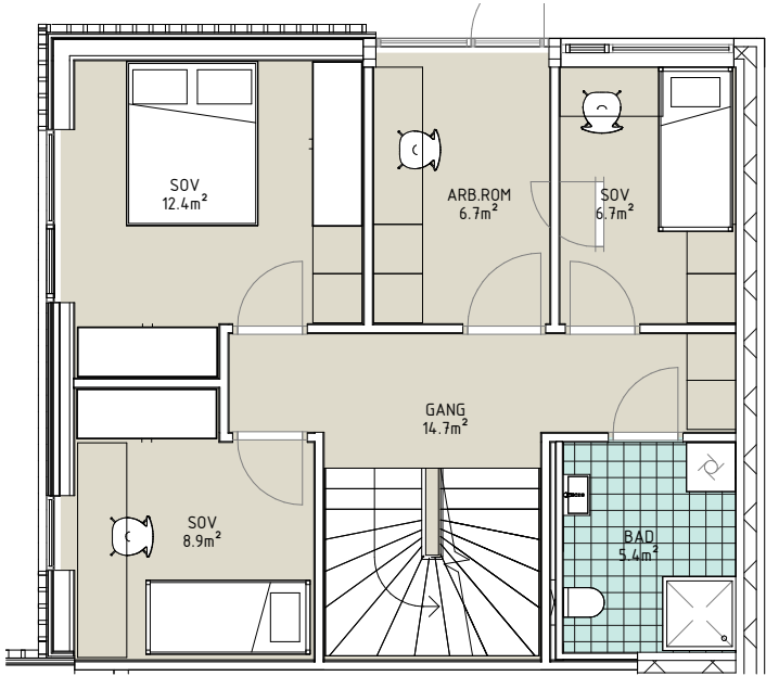
PLAN 1 1 : 100
