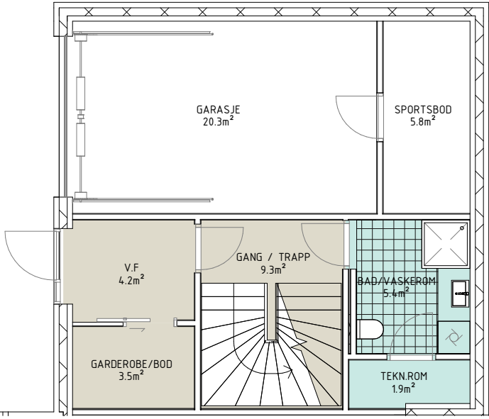
PLAN U 1 : 100
