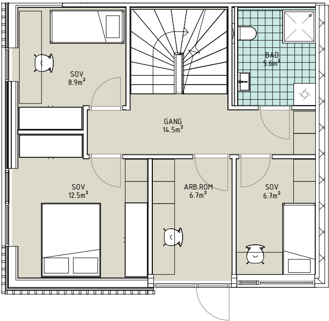
PLAN 1 1 : 100
