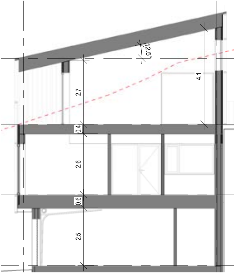
Snitt
