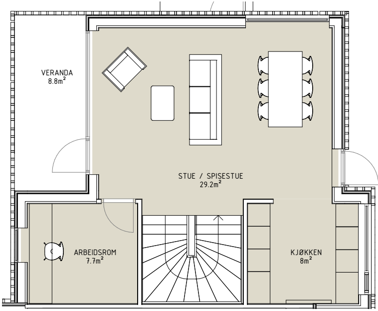
PLAN 2 1 : 100
