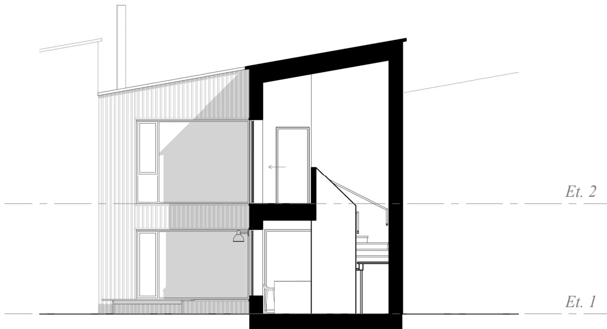
Fasade nord/vest (atrium)
