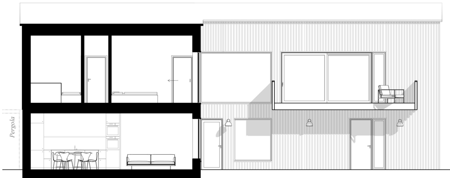
Fasade nord/øst (atrium)
