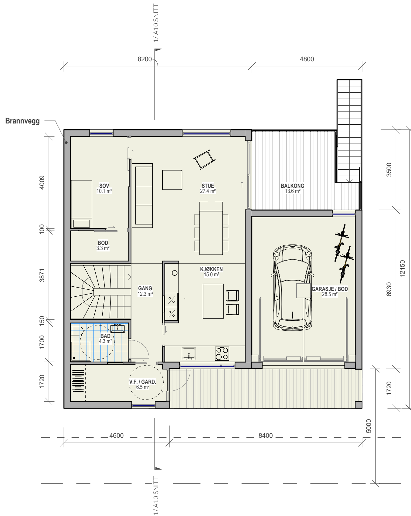
PLAN 1_HUS A2
