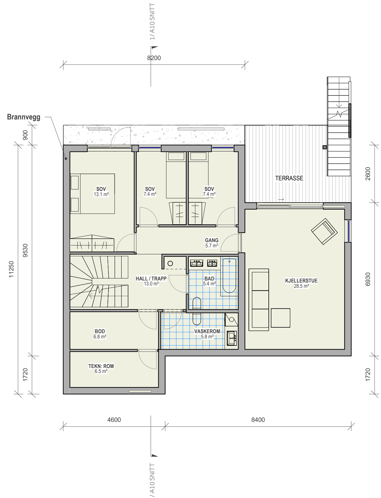
PLAN U_HUS A2
