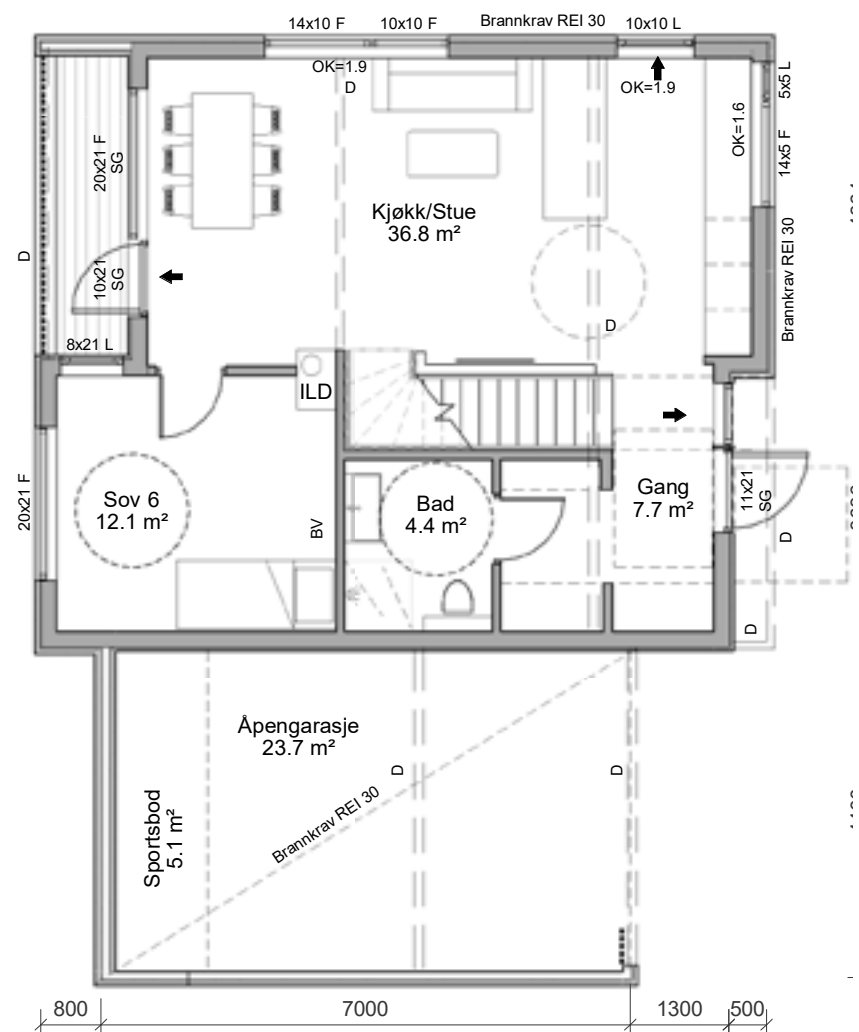
1. etasje
